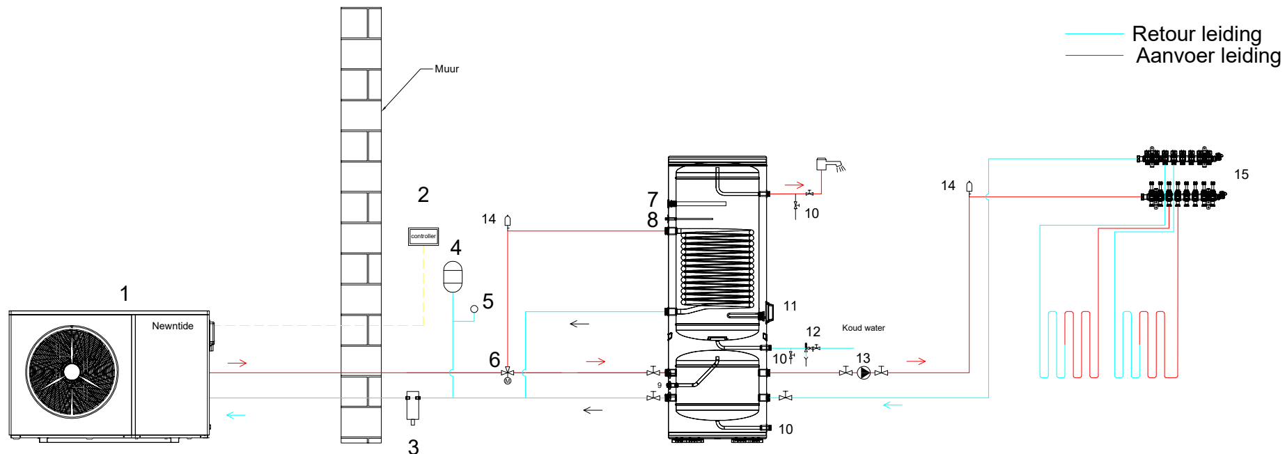
Installatieschema verwarmen/koelen + warm tapwater
